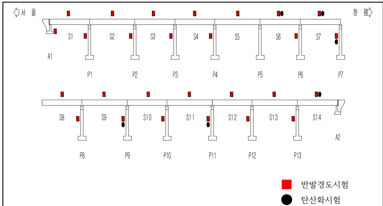
콘크리트 내구성조사 위치도
